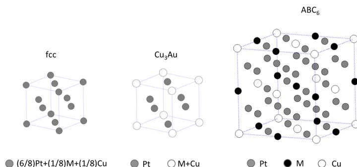
図 1: 2段階規則相転移における各相の構造.
