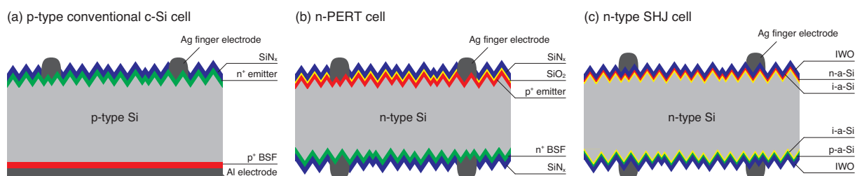
図 1: 各種太陽電池セルの断面構造. (a) p 型 c-Si セル, (b) n-PERT セル, および (c) n 型 SHJ セル. 図中の BSF, IWO はそれぞれ back surface field, W-doped \text{In}_2\text{O}_3 の略称である. また n-a-Si, i-a-Si, および p-a-Si はそれぞれ n 型, 真正, および p 型アモルファスシリコンを意味している.
